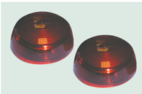
A.LR.470200.RO Remlicht, rood, Ø67 mm
